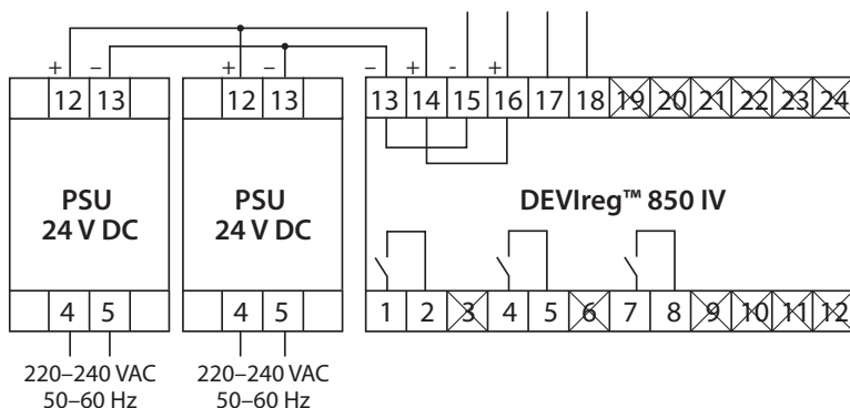
**Fig. H — Anschluß von 2 pcs. Netzteilen
