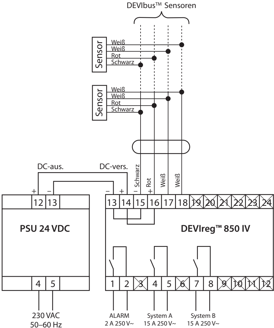
Fig. A — Anschlussplan DEVIreg™ 850 IV
